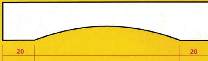
Linteau Cintre : Toute épaisseur / Flèche de 10 / Réf. Licte
