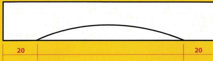
Linteau Cintre : Mi-épaisseur / Flèche de 10 / Réf. Licme
